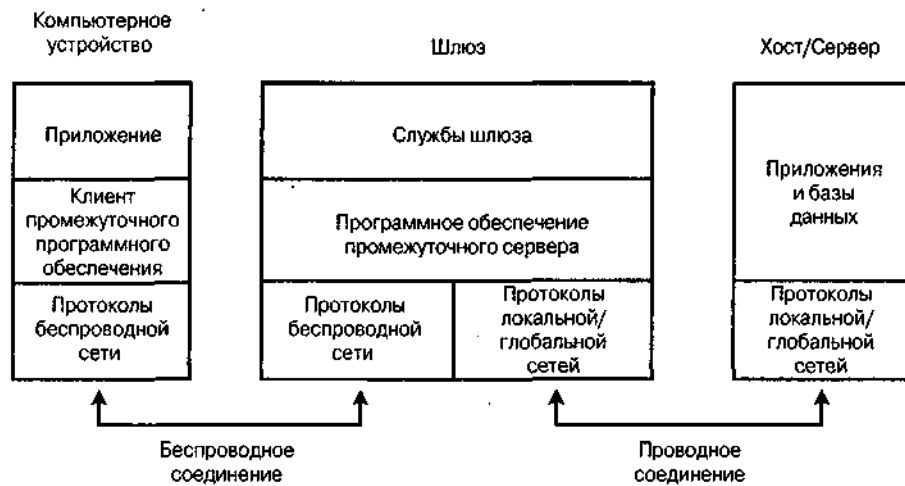
Рис. 2.5. Промежуточное программное обеспечение обеспечивает эффективное взаимодействие приложений компьютерных устройств с хостами и серверами
