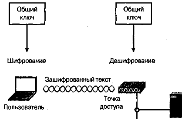
Рис. 8.4. При симметричном шифровании используется общий ключ
