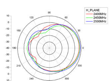
H-Plane
