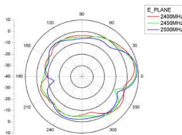
E-Plane
