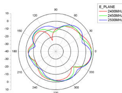
E-Plane
