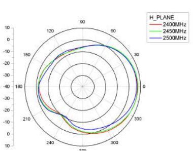
H-Plane
